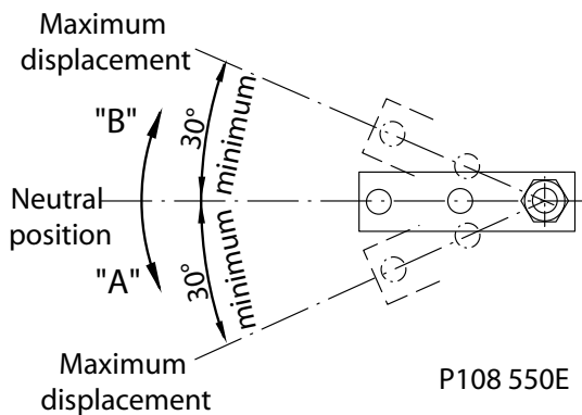
MDC handle rotation parameters
